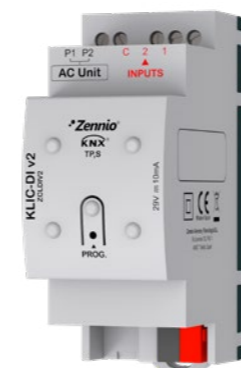
ZCLDIV2 (90 x 60 x 35 mm)
