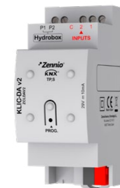
ZCLDAV2 (90 x 60 x 35 mm)
