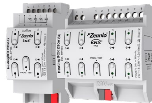
ZCL-4HT230 (90 x 60 x 35 mm) ZCL-8HT230 (90 x 60 x 80 mm)
